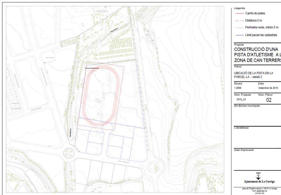
Estudi d'alternatives. Opció 2: pista a l'oest de la parcel·la
